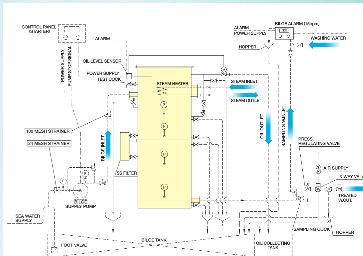
実線部はササクラの標準供給範囲を示します。 Solid lines indicate the standard piping fittings and accessories provided by Sasakura.
