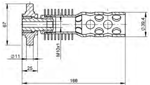
図 7: トムソンアダプタ 型式6513AK
